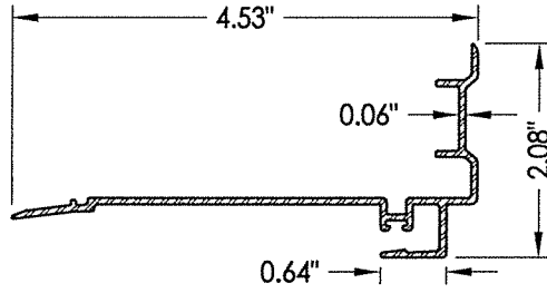
5 INTERLOCK 356-A54
