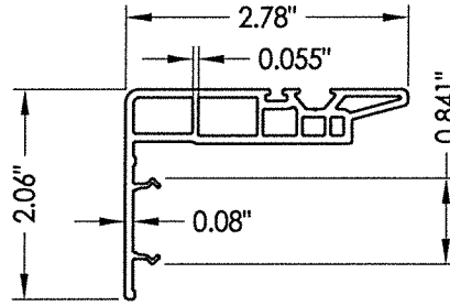
5 INTERLOCK 8573-356-D63
