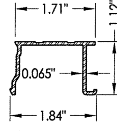
6 SILL CAP 356-A51-52-COV
